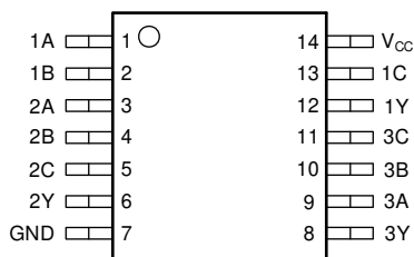
图 4-1. SN74AC10-Q1 PW 封装 ( 顶视图 )
