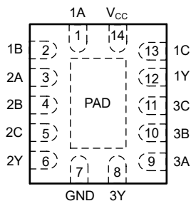
图 4-2. SN74AC10-Q1 BQA 封装 ( 顶视图 )
