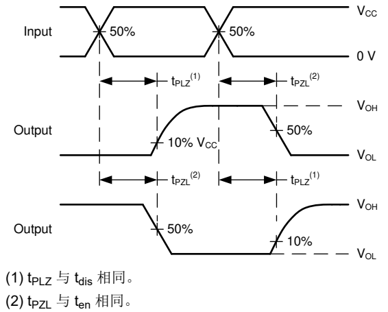
图 6-2. 电压波形传播延迟
