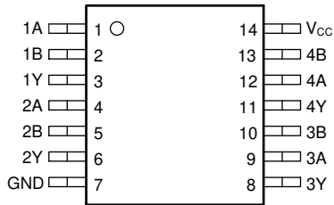
图 4-2. SN74AC09-Q1 、PW 封装 ( 顶视图 )
