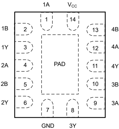
图 4-1. SN74AC09-Q1 BQA 封装 ( 顶视图 )
