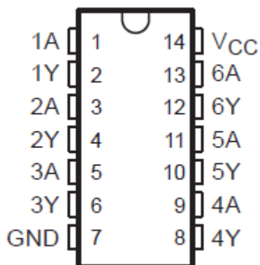
图 4-1. PW 封装，14 引脚 TSSOP (俯视图)
