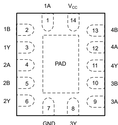
BQA 封装， 14 引脚 WQFN ( 透明顶视图 )
