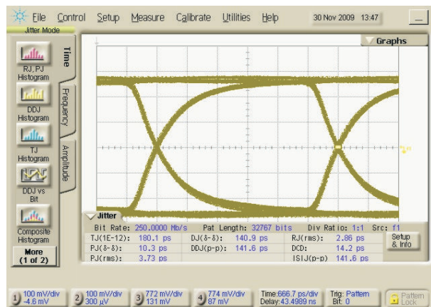
图 5-20. 驱动器输出眼图 250Mbps, 2^{15}-1 PRBS, V_{CC} = 3.3\text{V}
