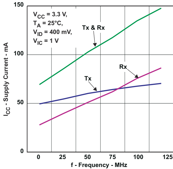
图 5-1. 电源电流与频率间的关系
