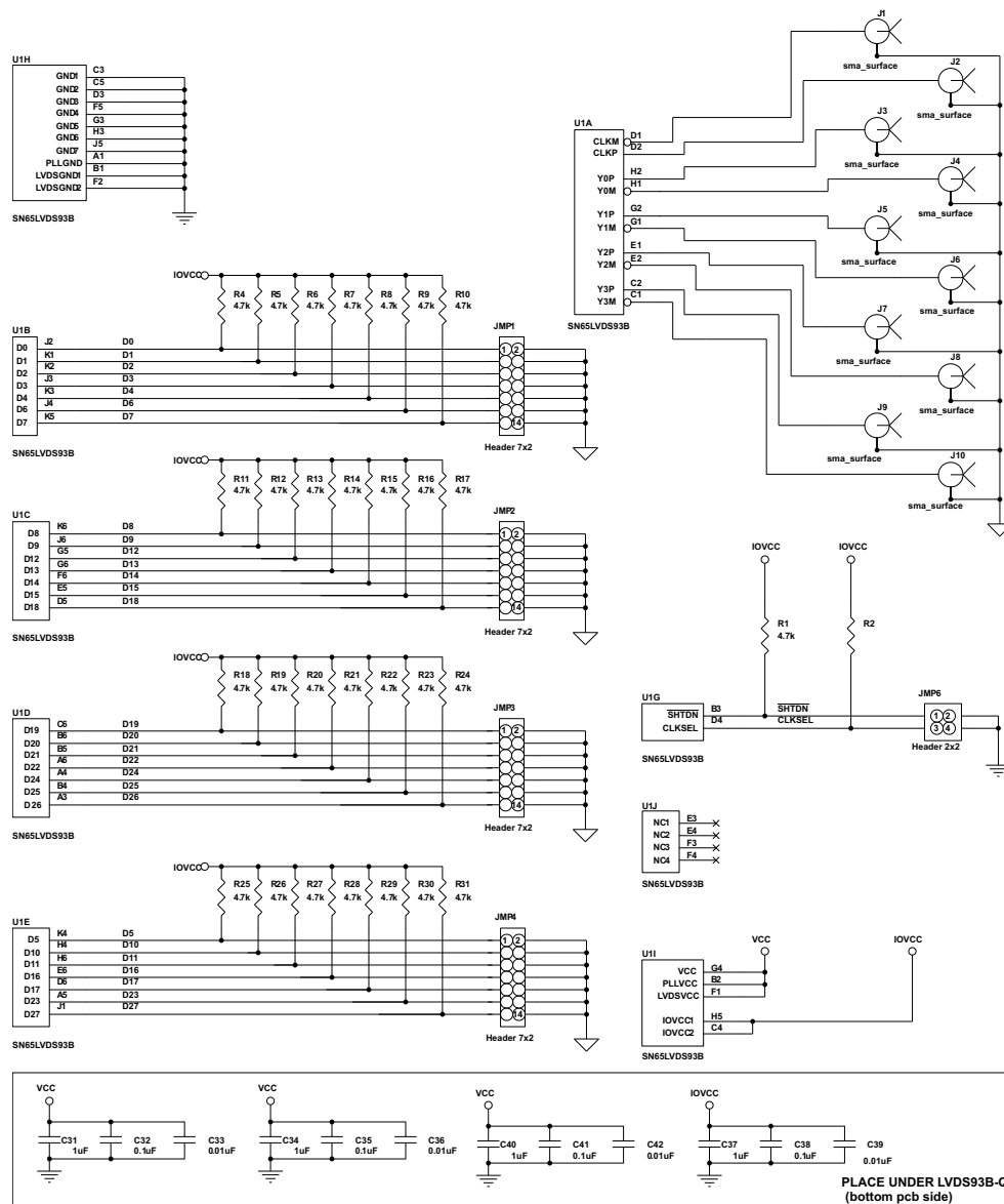
图 12. Schematic Example
