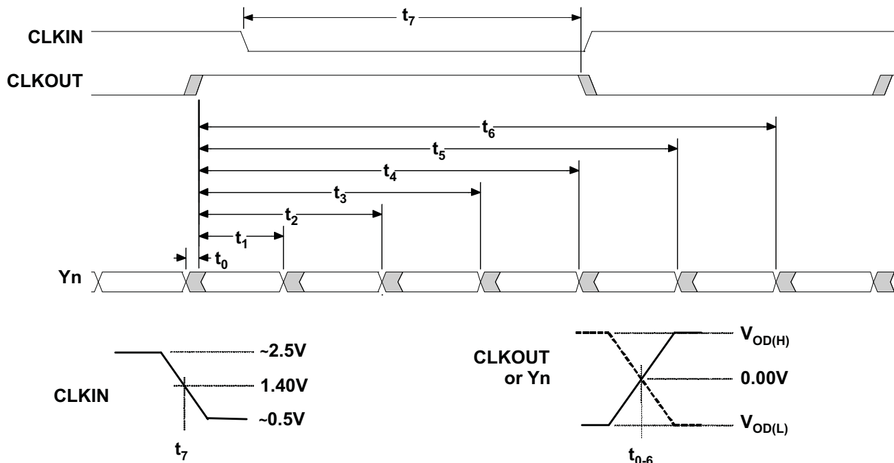
图 8. SN65LVDS93B-Q1 Timing Definitions
