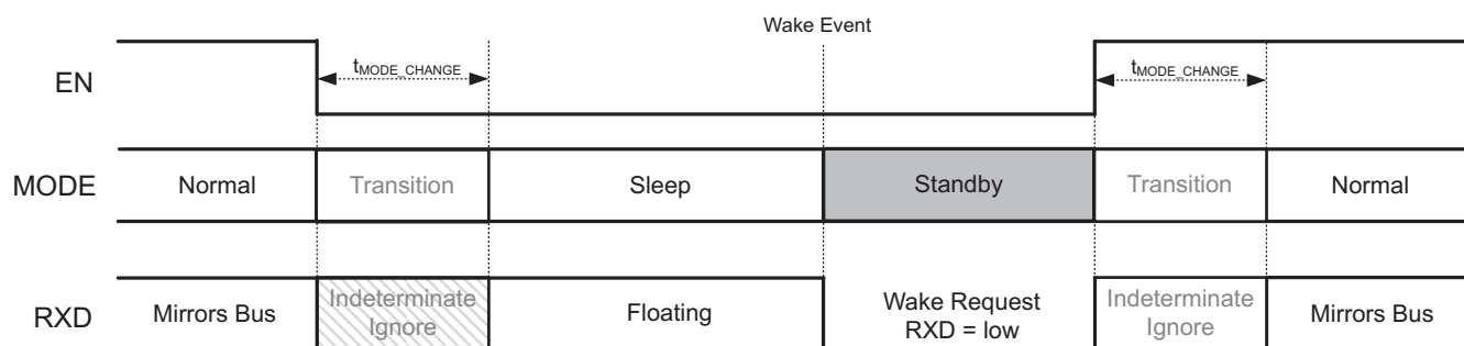
图 7-3. Mode Transitions
