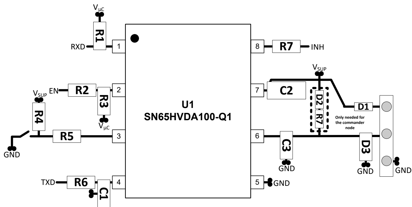
图 12-1. Layout Schematic
