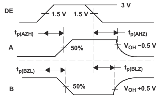
图 7-7. Driver Enable/Disable Test
