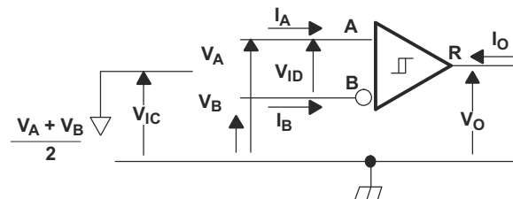
图 7-9. Receiver DC Parameter Definitions
