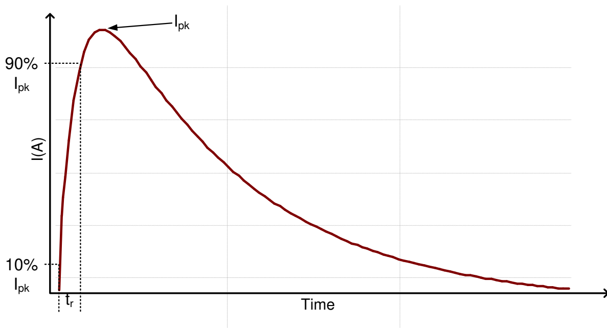
图 10-2. HBM Curve
