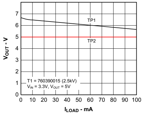
图 6-11. Output Voltage vs Load Current
