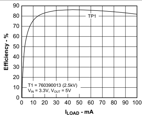
图 6-6. Efficiency vs Load Current
