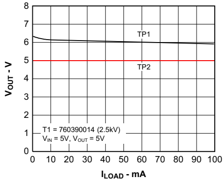
图 6-9. Output Voltage vs Load Current
