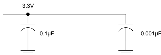
图 9-1. 建议的 LVDS 旁路电容器布局
