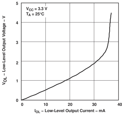
图 5-1. 低电平输出电压与低电平输出电流间的关系
