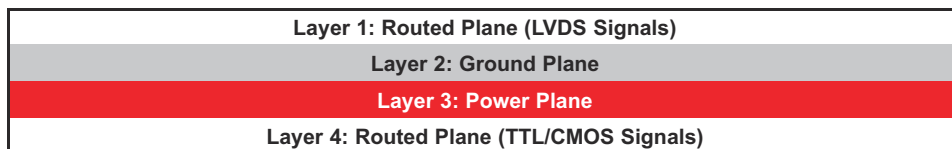
图 10-3. 四层 PCB 板
