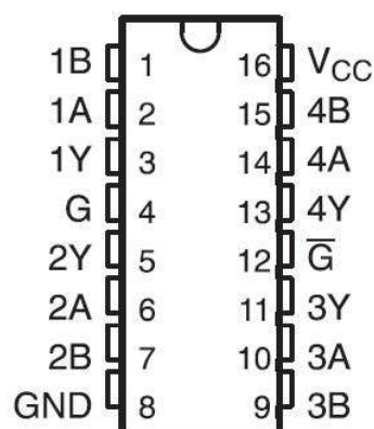
图 4-1. D 封装，16 引脚，SOIC ( 顶视图 )
