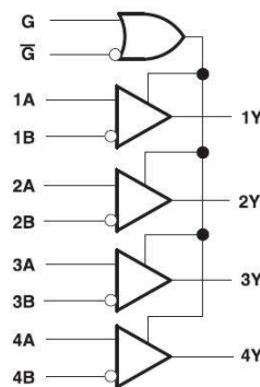
逻辑图 ( 正逻辑 )
