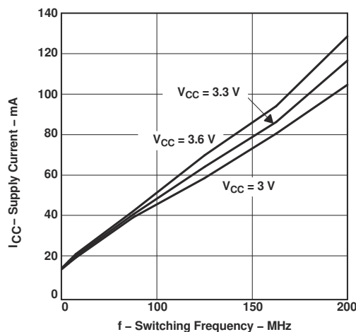
图 5-5. 电源电流与频率间的关系
