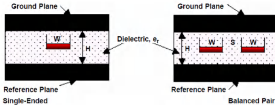
图 10-2. 带状线拓扑
