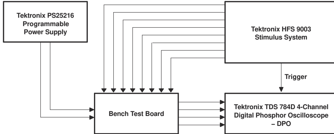
图 8-6. 设备设置
