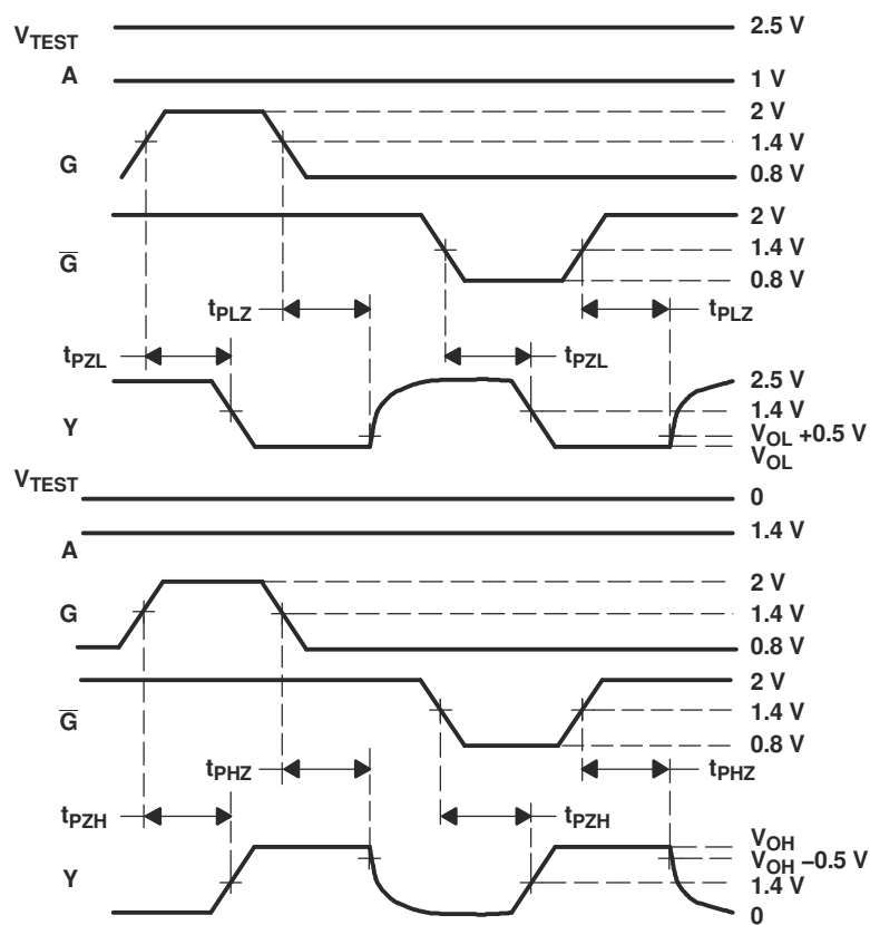
图 6-4. 启用/禁用时间测试电路和波形
