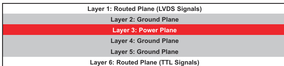
图 10-4. 六层 PCB 板
