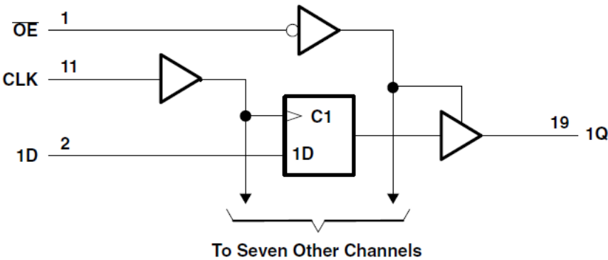
图 7-4. 逻辑图（正逻辑）
