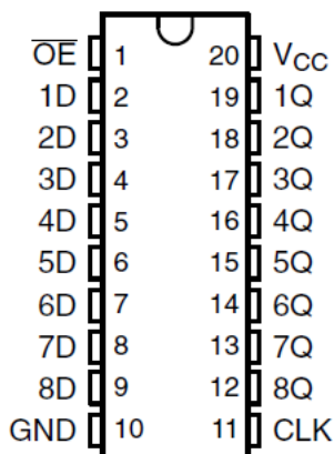
图 4-1. PW 封装 ( 顶视图 )
