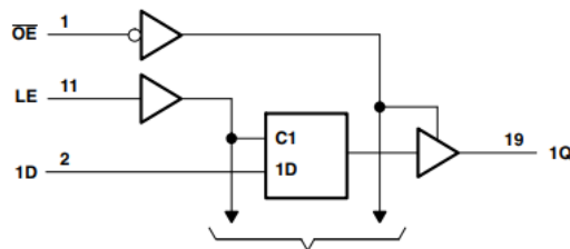
图 7-1. 逻辑图（正逻辑）
