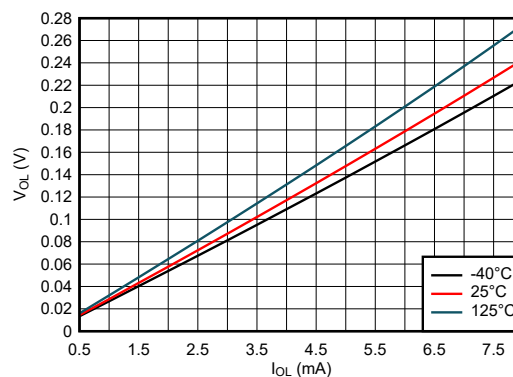
图 5-12. 低电平状态下输出电压与电流间的关系 (1.8V 电源)
