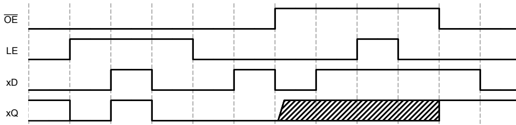
图 8-2. 应用时序图
