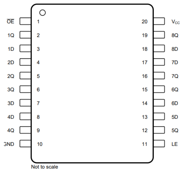
图 4-1. PW 20 引脚 TSSOP ( 顶视图 )
