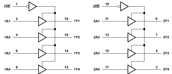
逻辑图 (正逻辑)
