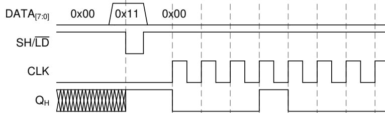
图 8-2. 应用时序图
