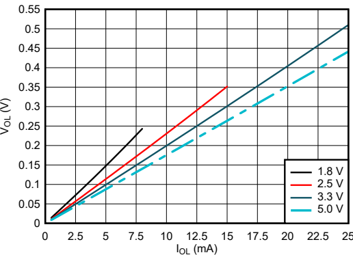
图 5-5. 低电平状态下输出电压与电流间的关系
