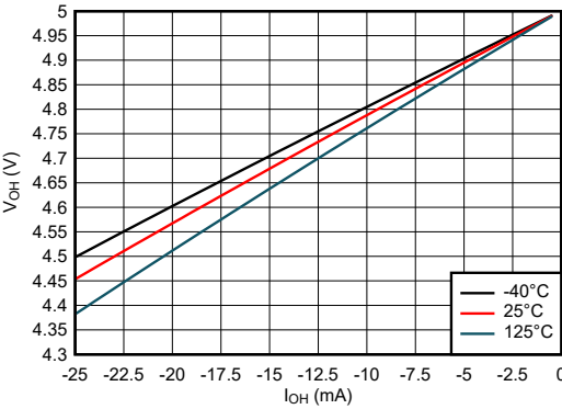
图 5-6. 高电平状态下输出电压与电流间的关系（5V 电源）
