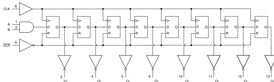
逻辑图 (正逻辑)
