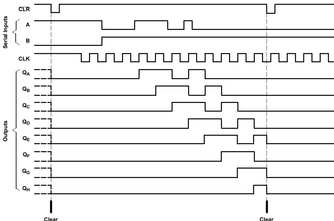
图 7-2. 应用时序图
