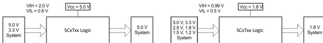
图 6-2. SCxT 升压和降压转换示例
