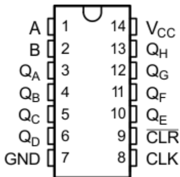
图 4-1. PW 封装 14 引脚 TSSOP (顶视图)
