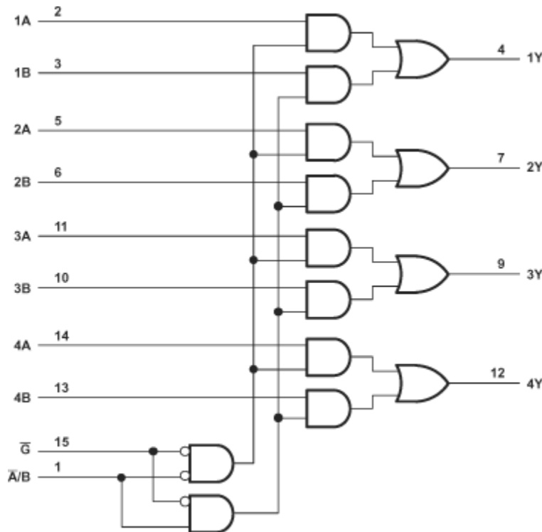
图 7-1. 逻辑图 (正逻辑)
