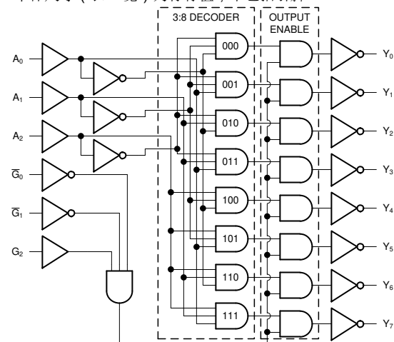
简化逻辑图 (正逻辑)
