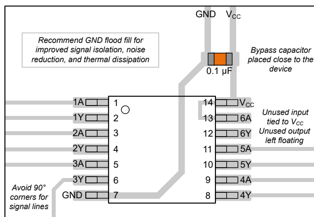
图 8-3. 示例布局 SN54SC6T17-SEP
