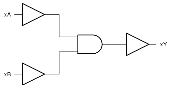
简化逻辑图
