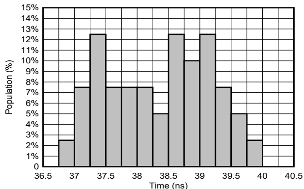
图 6-14. T_{PD} 分布；1.2V； T_A = -55^\circ\text{C} 至 125^\circ\text{C} (40 个样本)
