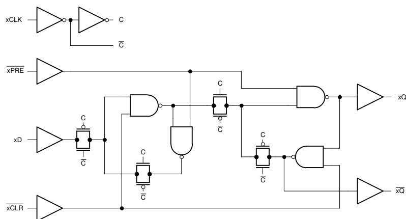
简化逻辑图
