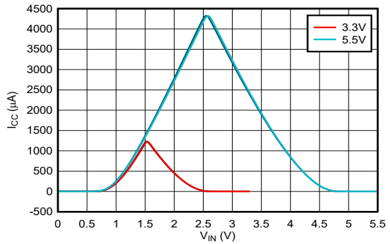
图 5-2. 电源电流与输入电源电压 ( 3.3V 至 5.5V ) 间的关系
