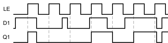
图 7-2. 应用时序图
