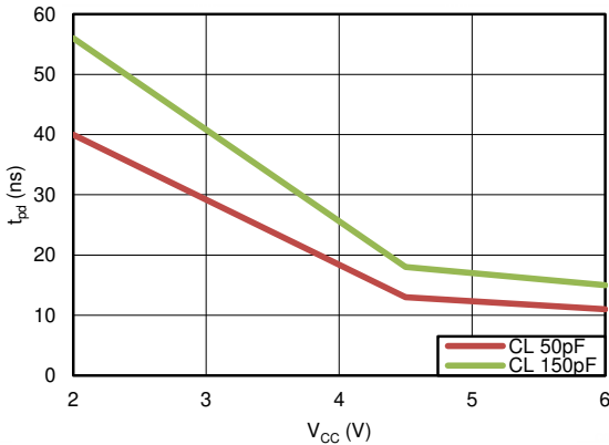
图 5-1. 传播延迟
