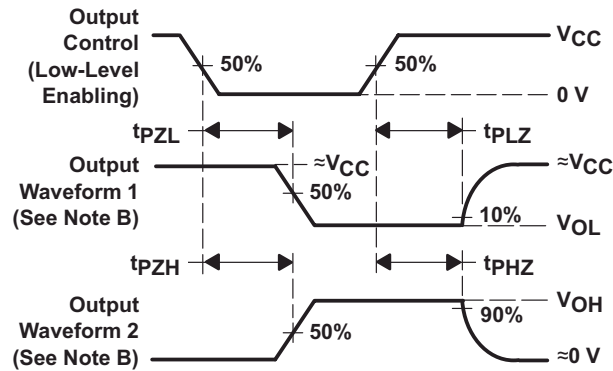
图 6-4. 三态输出的 启用和禁用时间
