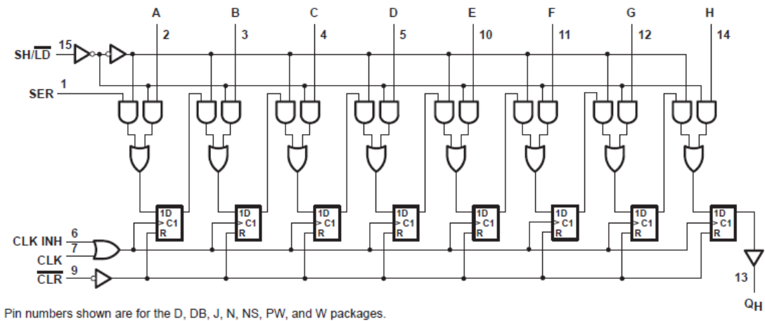
功能方框图
