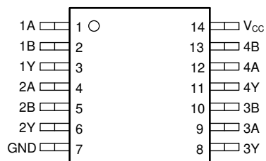
D、DB、N、PW、J 或 W 封装
