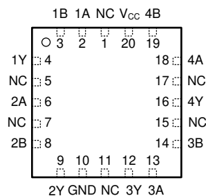
FK 封装
