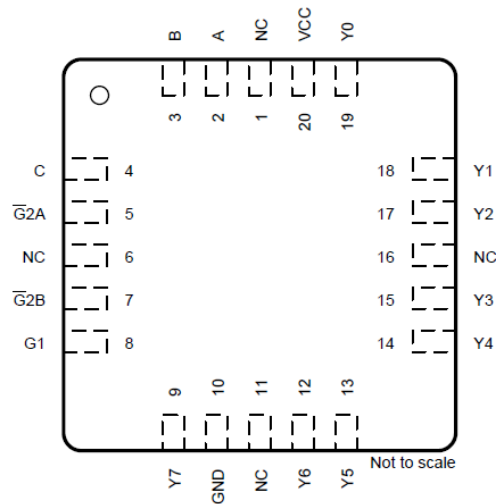
图 3-3. FK 封装， 20 引脚 LCCC (顶视图)
