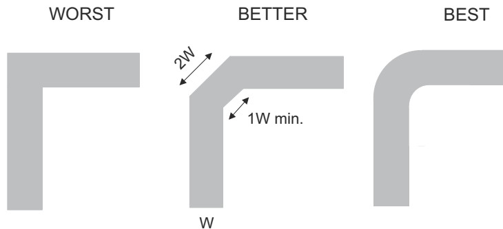
图 8-5. 布线示例
