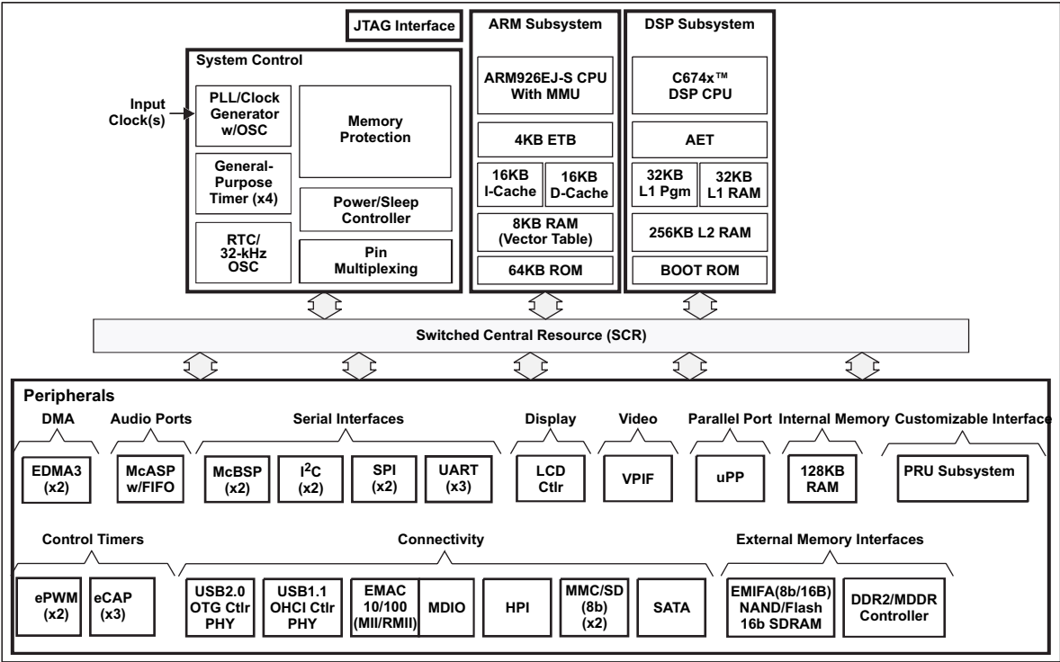
图 1-1. 功能方框图
