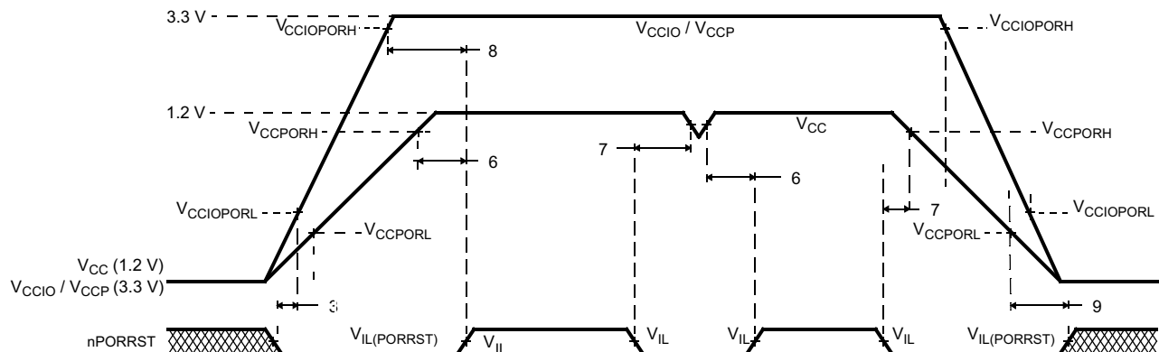
图 6-1. nPORRST Timing Diagram (A)
