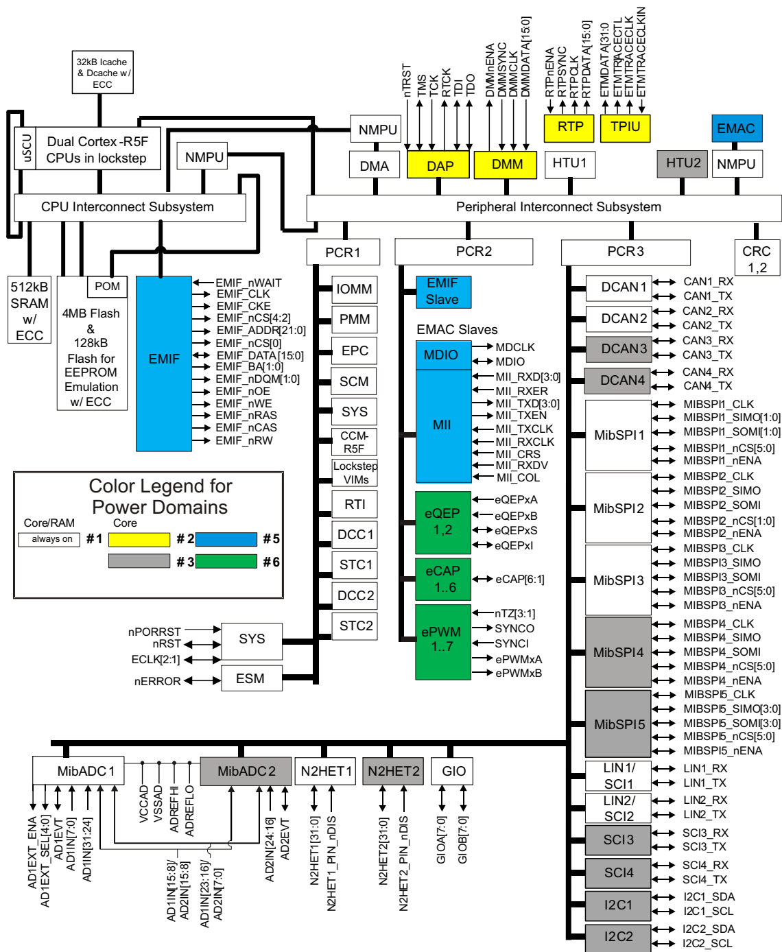
图 1-1. 功能方框图
