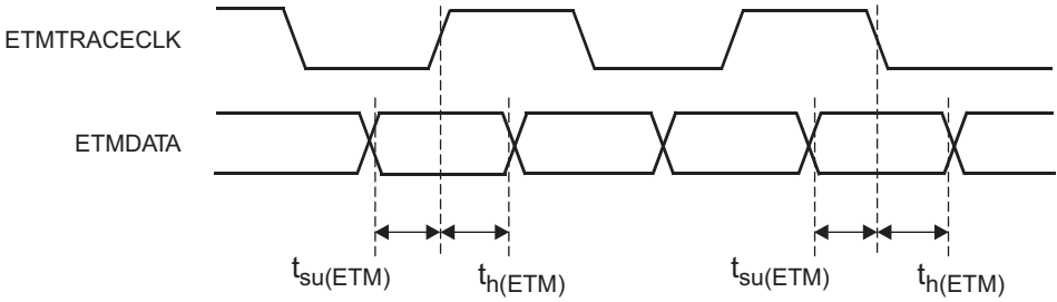
图 6-31. ETMDATA Timing
