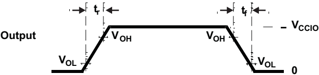
图 5-3. CMOS-Level Outputs
