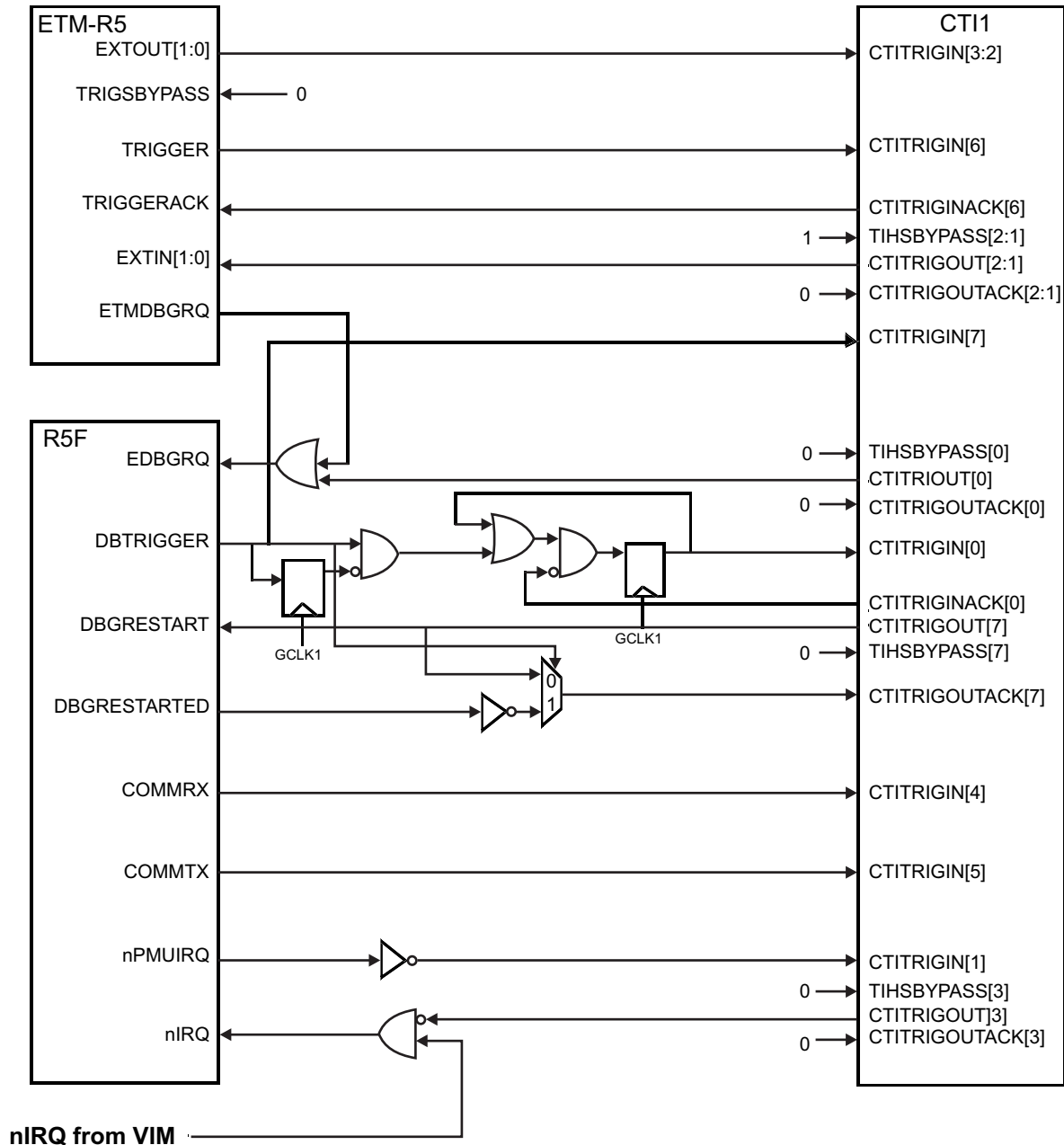
图 6-25. CTI1 Mapping
