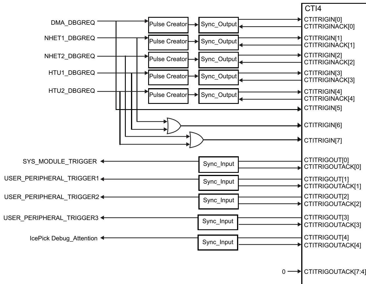
图 6-27. CTI4 Mapping
