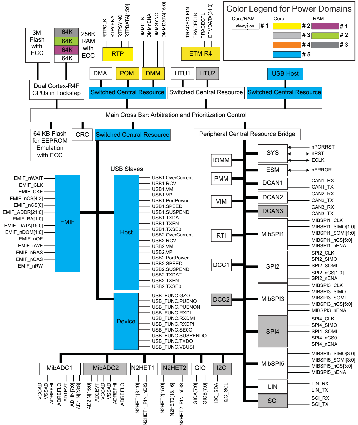
图 1-1. 功能方框图
