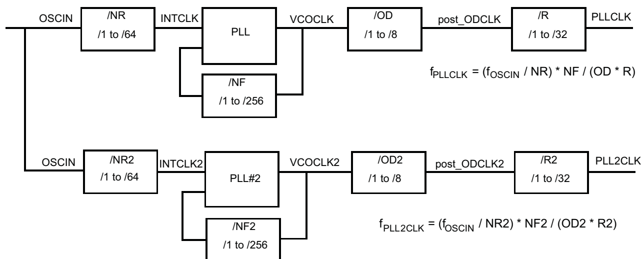
图 5-6. PLLx 方框图
