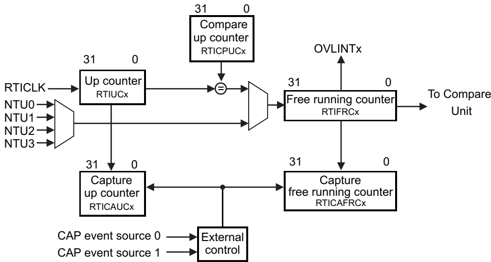
图 5-18. 计数器块图
