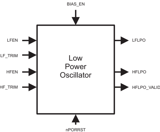
图 5-5. LPO 方框图
