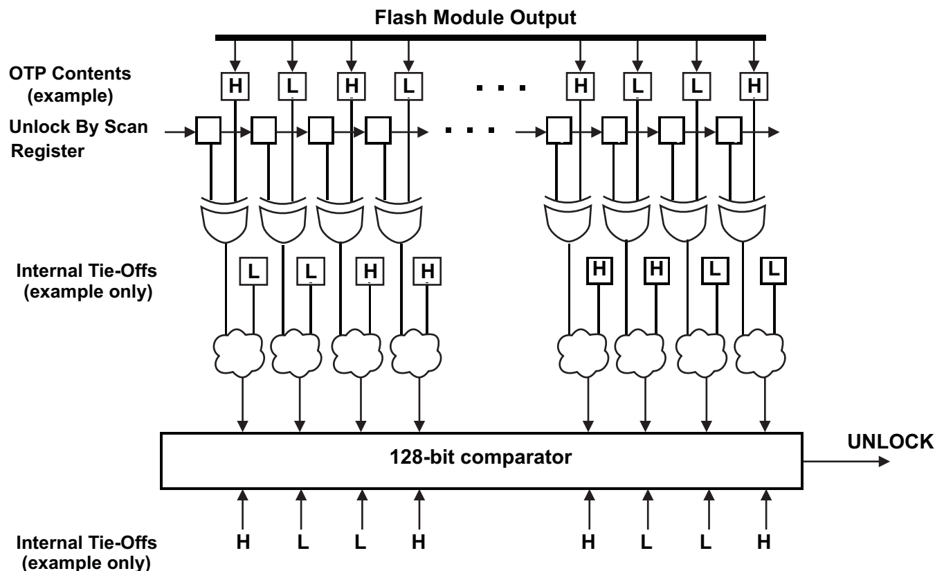
图 5-21. AJSM 解锁
