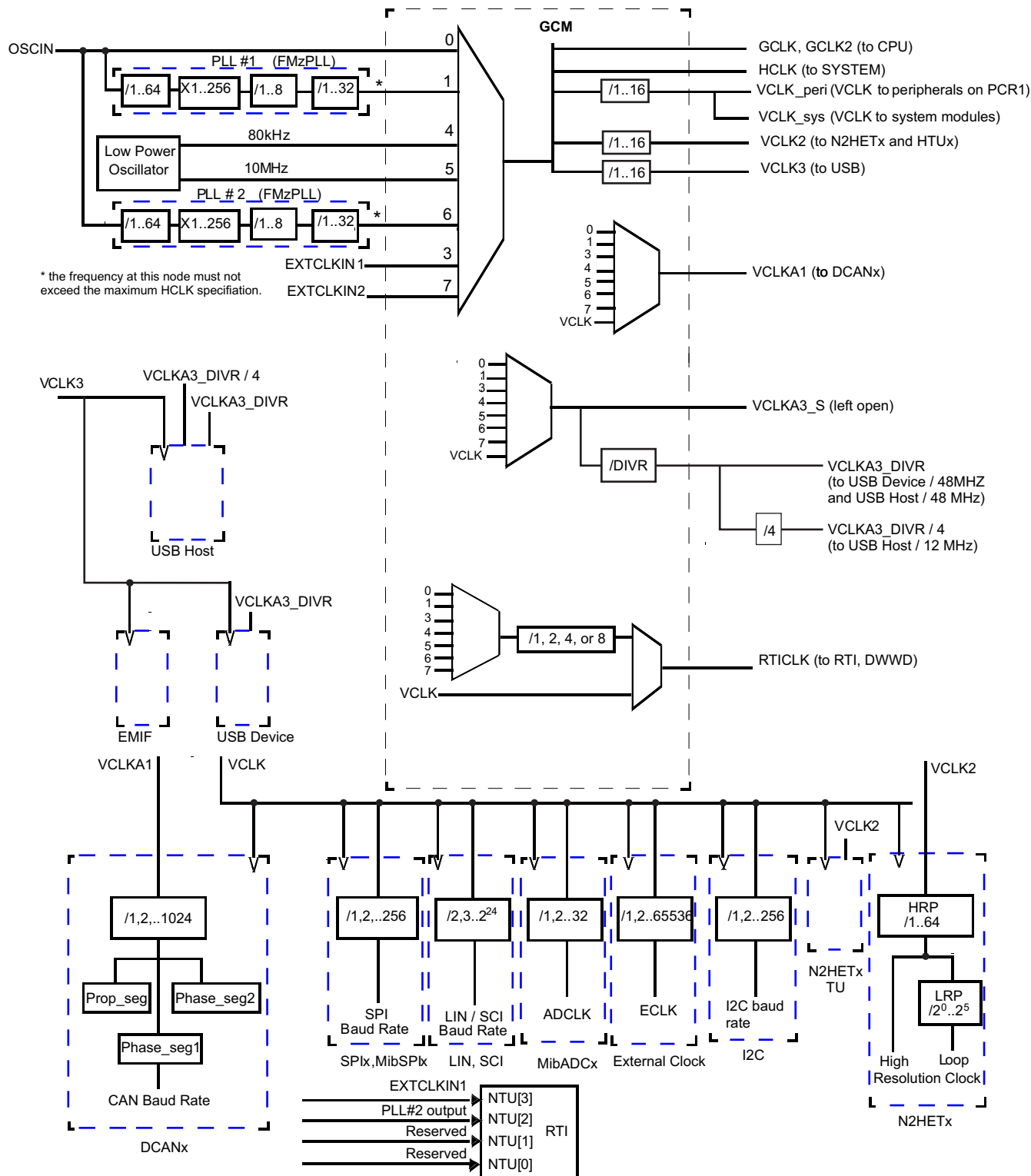
图 5-7. 器件时钟域
