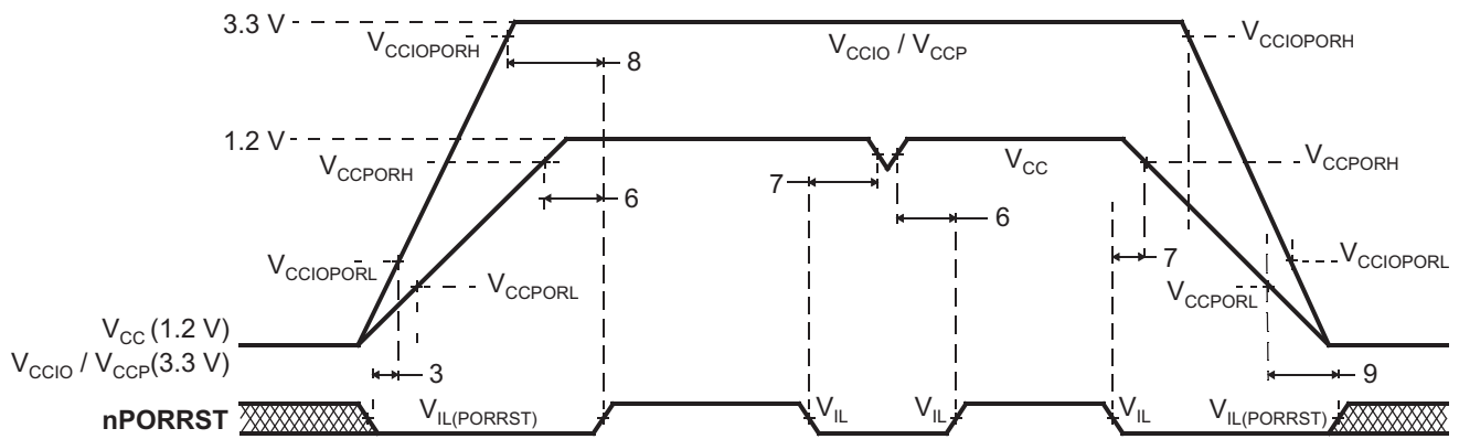
图 5-1. nPORRST 时序图
