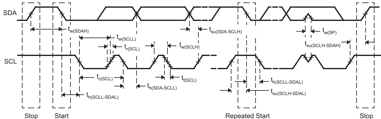
图 6-13. I2C 时序
