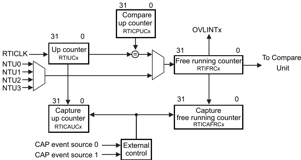
图 5-17. 计数器块图
