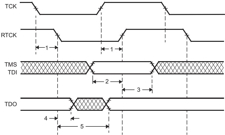
图 5-20. JTAG 时序
