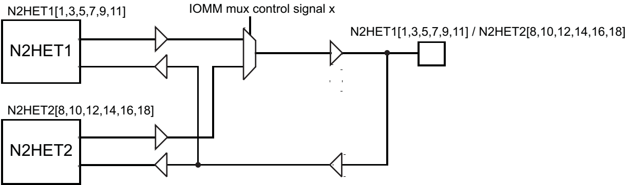
图 6-12. N2HET 监视
