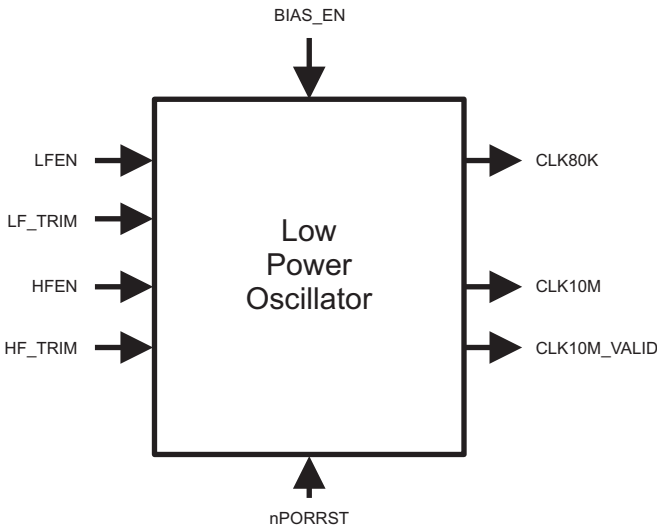
图 4-5. LPO 方框图
