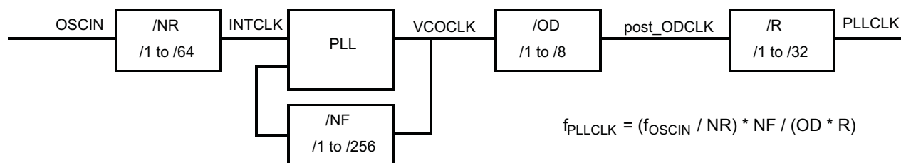
图 4-6. PLL 方框图
