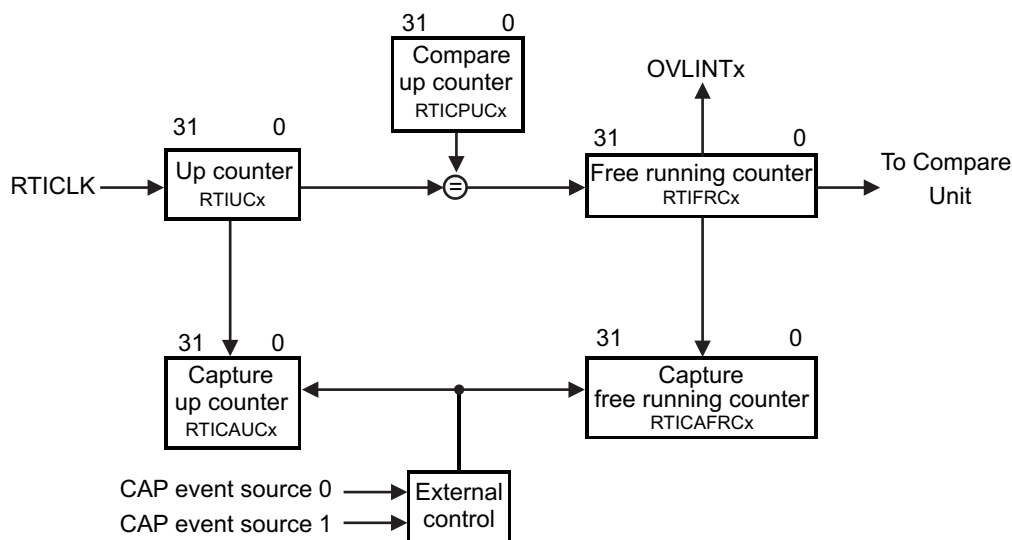
图 4-11. 计数器块图
