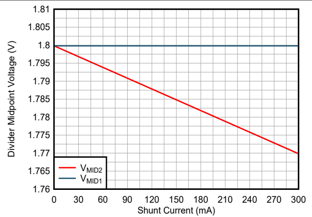
图 8-10. VMID 的仿真结果
