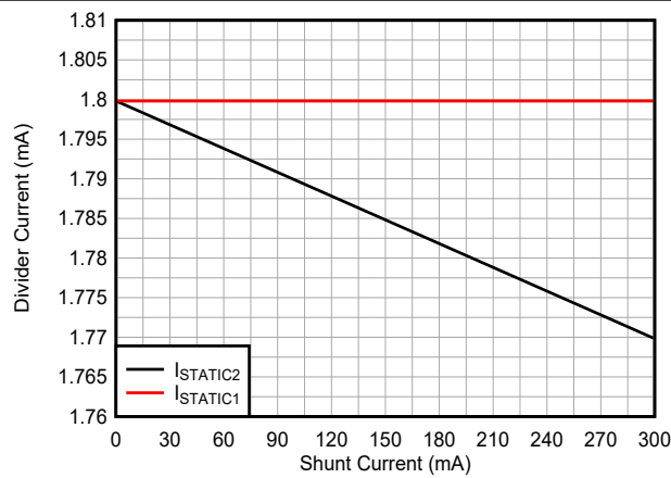
图 8-9. ISTATIC 的仿真结果
