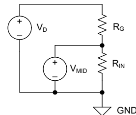
图 6-3. 分压器电路
