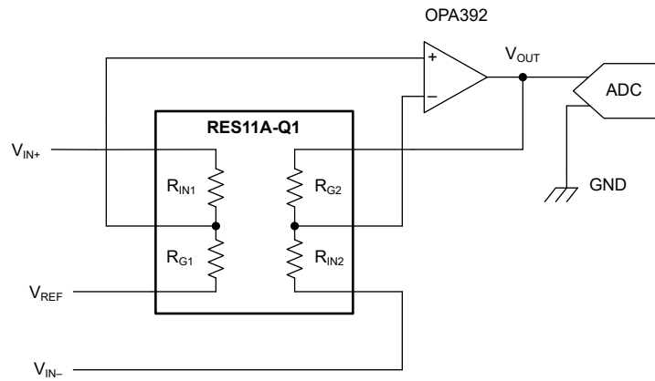
图 8-1. 使用 RES11A-Q1 的分立式差分放大器
