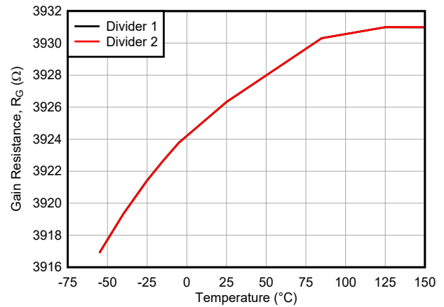
图 5-8. R_{Gx} 与温度间的关系
