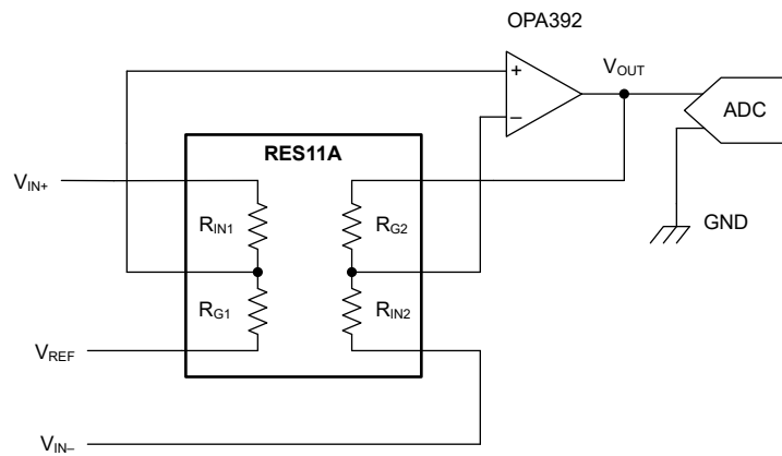
图 8-1. 使用 RES11A 的分立式差分放大器
