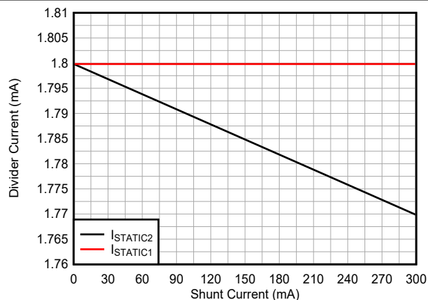
图 8-9. I STATIC 的仿真结果
