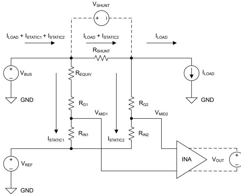
图 8-6. RES11A 共模转换电路
