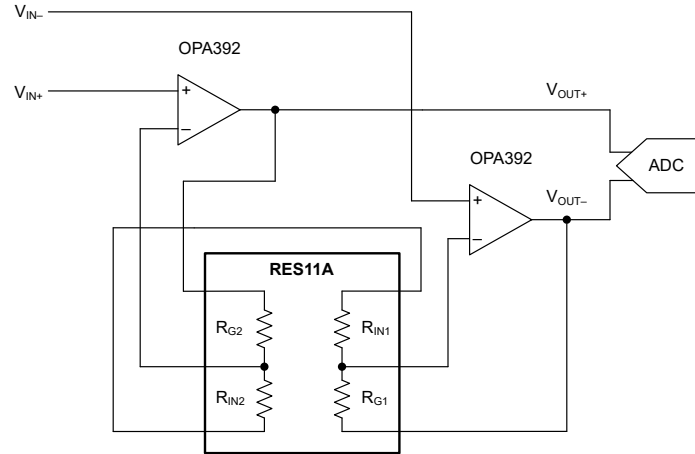
图 8-3. 使用 RES11A 的差分输入、差分输出仪表放大器
