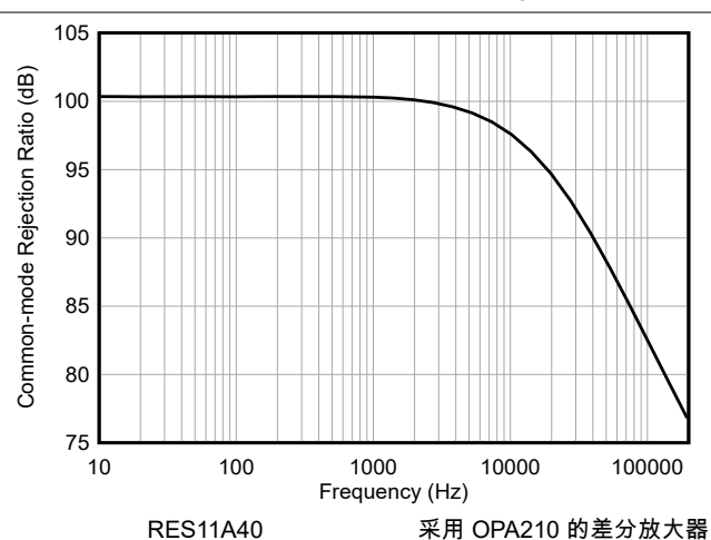
图 5-24. CMRR 与频率之间的关系
