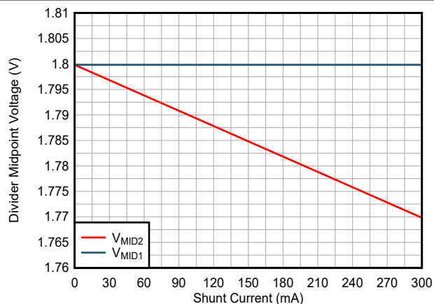
图 8-10. VMID 的仿真结果
