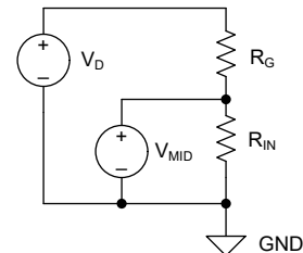
图 6-3. 分压器电路
