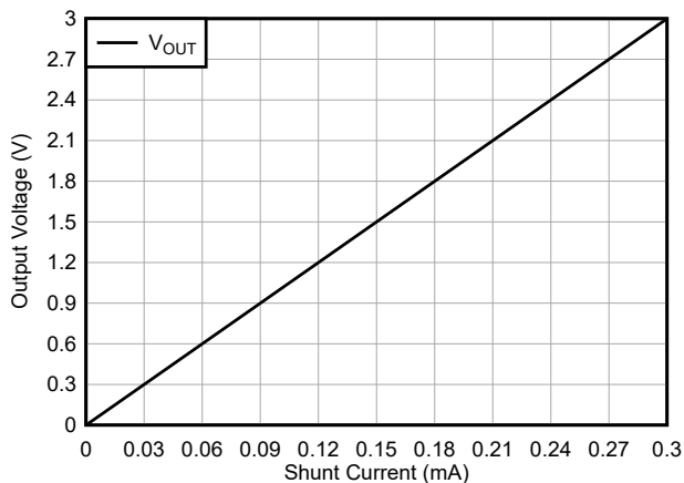
图 8-11. VOUT 的仿真结果
