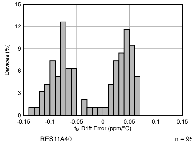
图 5-14. t_M 漂移分布
