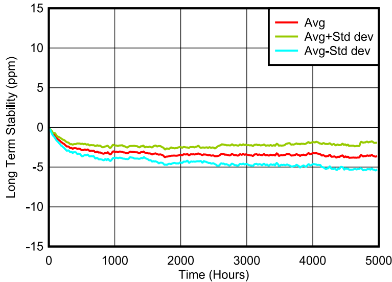
图 8-1. 长期稳定性( V_{REF\_Z} )
