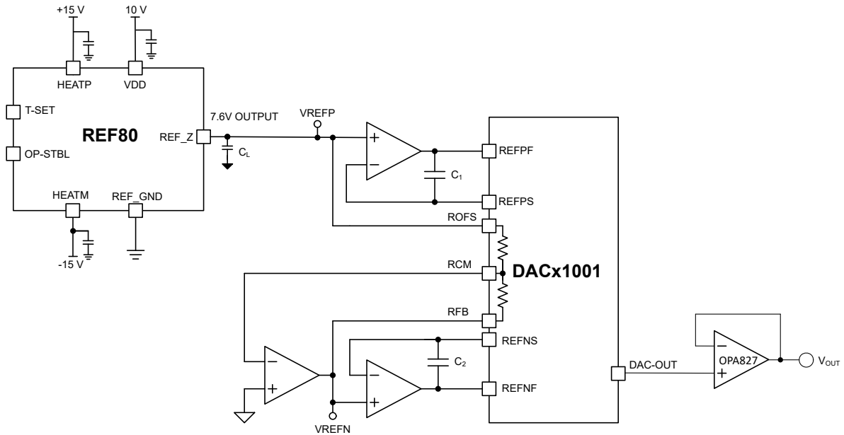
图 9-5. 使用 DACx1001 的精密信号
