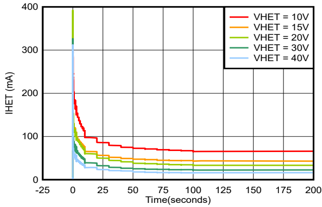
图 6-7. 启动加热器电流 IHET 与时间间的关系
