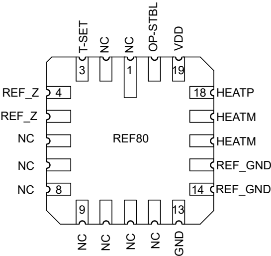
图 5-1. NAJ 封装 20 引脚 LCCC 顶视图
