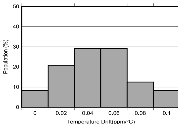
图 8-3. 漂移分布
