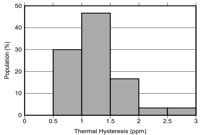
图 6-12. 热迟滞 (周期 1) 分布 T_A = 0^\circ\text{C} 至 70^\circ\text{C}
