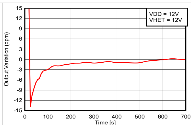
图 6-14. 启动行为
