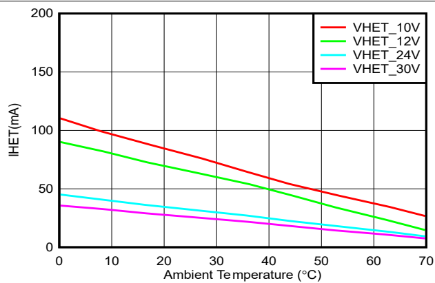
图 6-6. 稳态加热器电流 I_{HET} 与温度间的关系
