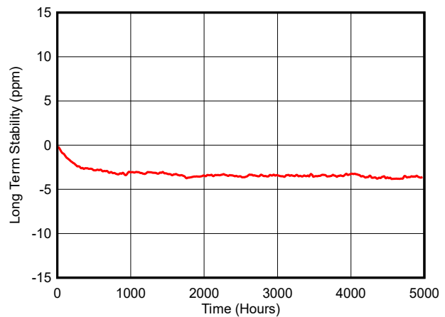
基准电压漂移与时间的关系
