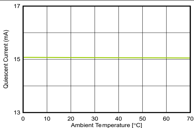
图 6-5. 电源电流 ( I_{VDD} ) 与温度间的关系
