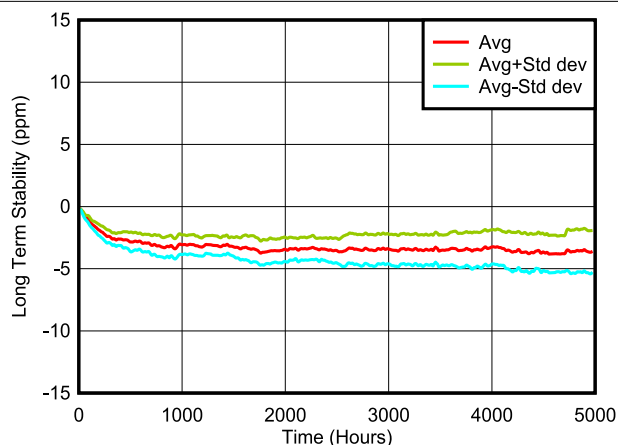
图 6-1. 长期稳定性
