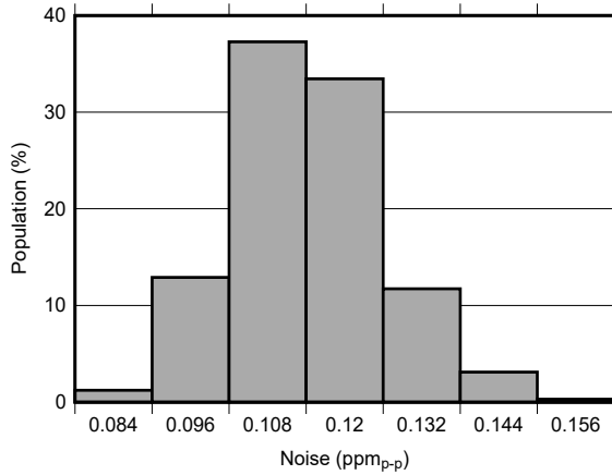
图 6-9. 0.1Hz 至 10Hz 电压噪声分布
