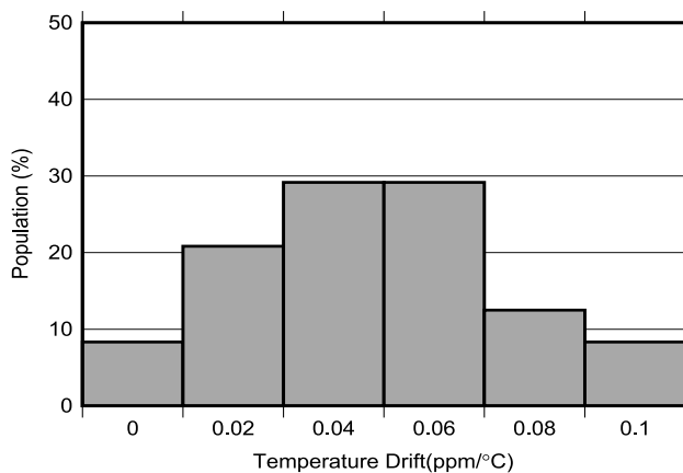
图 6-3. 漂移分布
