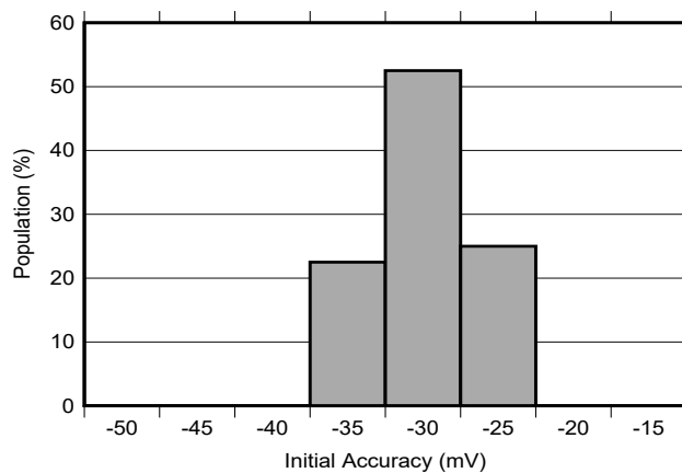
图 6-4. 精度分布
