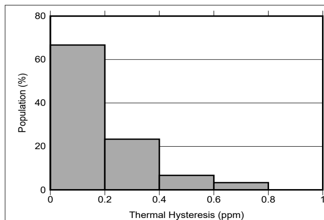
图 6-13. 热迟滞 (周期 2) 分布 T_A = 0^\circ\text{C} 至 70^\circ\text{C}
