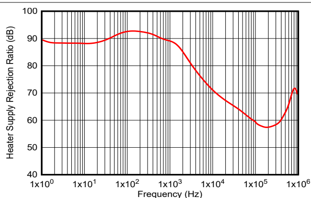
图 6-16. 加热器电源抑制比与频率间的关系
