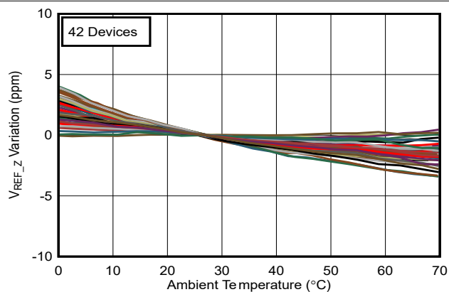
图 6-2. V_{REF\_Z} 与自然通风温度间的关系
