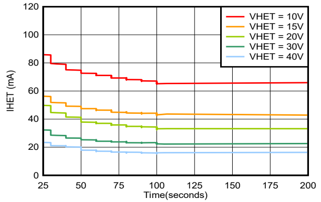
图 6-8. 启动加热器电流 (放大图) IHET 与时间间的关系
