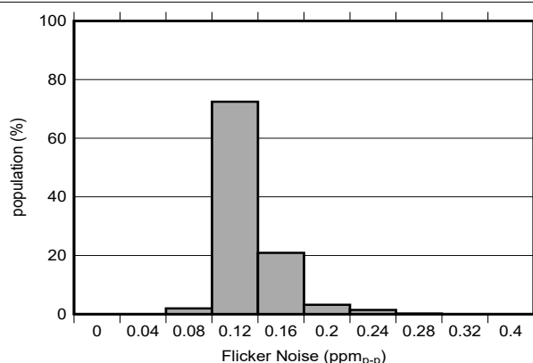
图 7-5. 0.1Hz 至 10Hz 电压噪声 (C NR = 100 μF)
