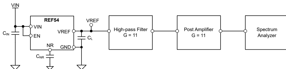
图 7-7. 宽带噪声测试设置
