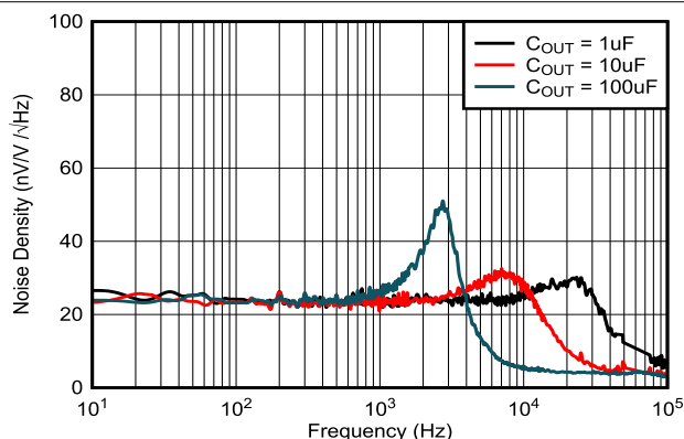
图 7-8. 噪声性能 10Hz 至 100kHz ( C_{NR} = 开路)
