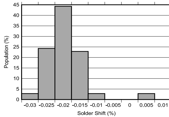
图 7-13. 焊接漂移
