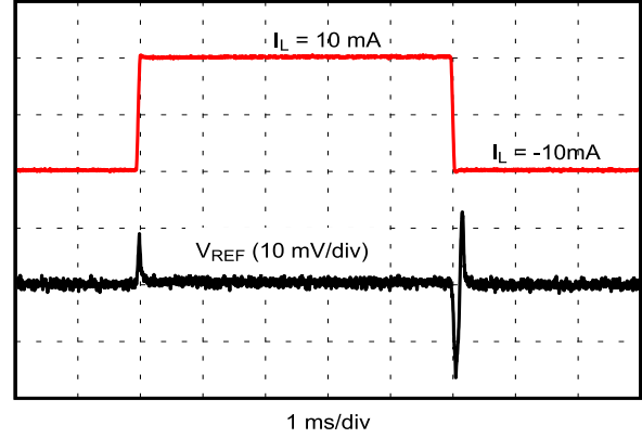
图 6-8. 负载瞬态响应 ( C_{OUT} = 10\text{ }\mu\text{F} )
