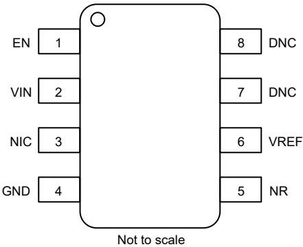
图 5-1. D 封装 8 引脚 SOIC 顶视图
