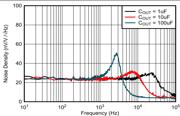
图 6-15. 噪声性能 10Hz 至 100kHz ( C_{NR} = \text{开路} )
