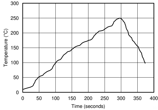
图 7-12. 回流焊曲线
