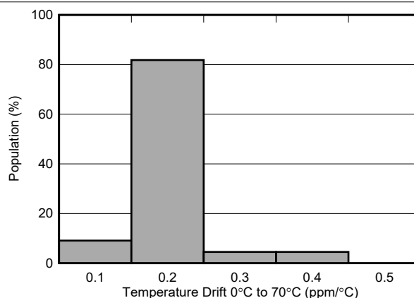
图 6-2. 漂移分布
