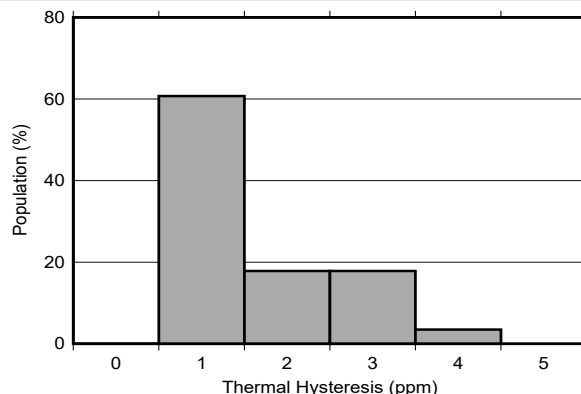
图 7-11. 热迟滞分布 ( 0^\circ\text{C} 至 70^\circ\text{C} ) - 周期 2 (REF54250CDR)
