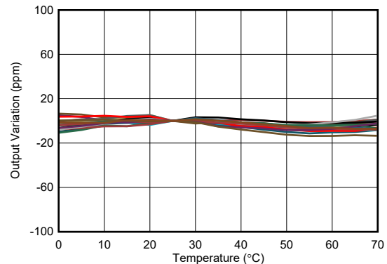
输出电压与自然通风温度间的关系
