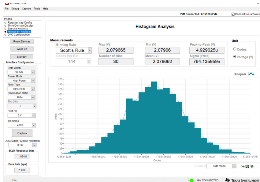
图 9-6. 使用 ADS1285 进行直流测量 ( VIN = 2.0796V ( 接近 FSR ) )
