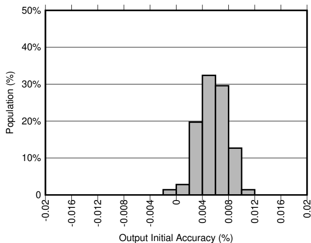
图 6-3. 精度分布
