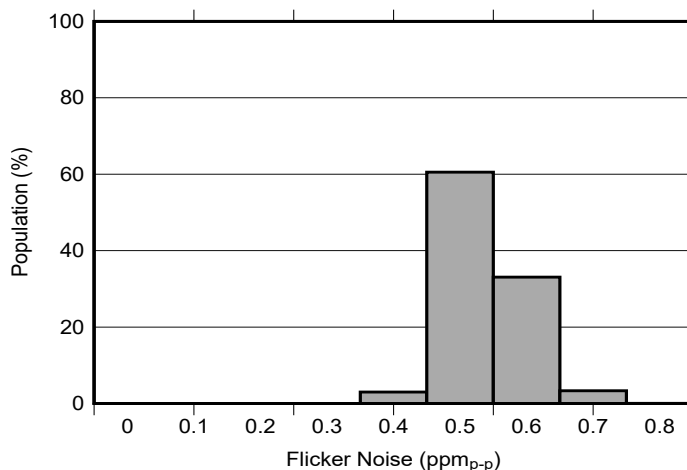
图 7-4. 0.1Hz 至 10Hz 电压噪声分布 (C NR = 开路)
