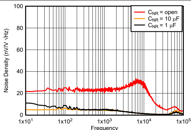
图 7-9. 噪声性能 10Hz 至 100kHz ( C_{OUT} ) = 10\ \mu\text{F}
