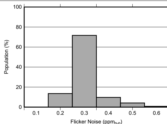
图 7-6. 0.1Hz 至 10Hz 电压噪声 (C NR = 10 μF)
