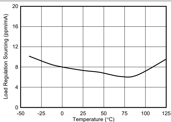
图 6-5. 负载调整率 (拉电流) 与温度间的关系
