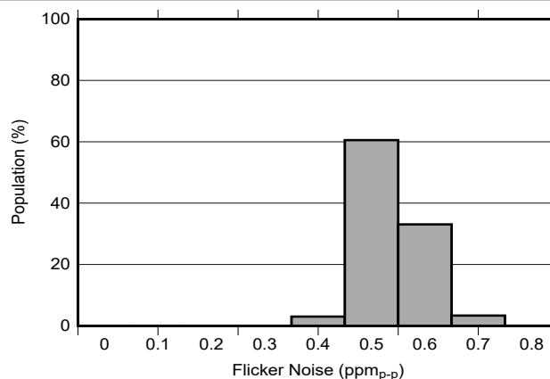
图 6-14. 0.1Hz 至 10Hz 电压噪声分布 ( C_{NR} = \text{开路} )
