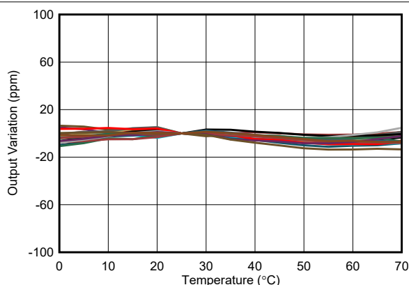
图 6-1. C 级输出电压与自然通风温度间的关系
