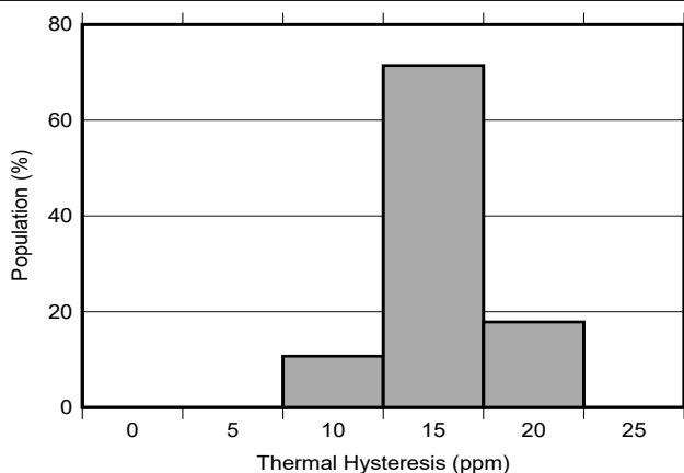
图 6-17. REF54250 热迟滞分布 ( 0^\circ\text{C} 至 70^\circ\text{C} )
