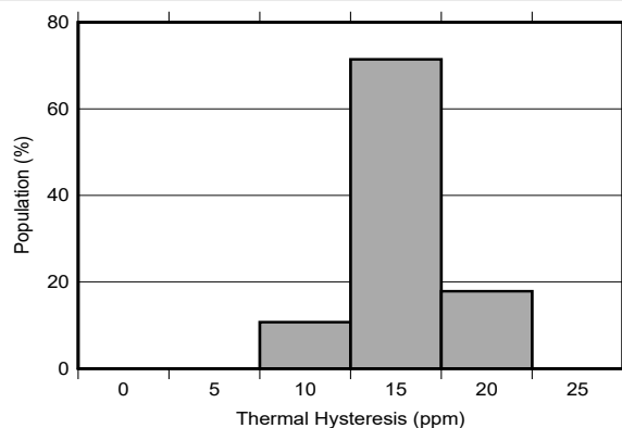
图 7-10. 热迟滞分布 ( 0^\circ\text{C} 至 70^\circ\text{C} ) - 周期 1 (REF54250CDR)
