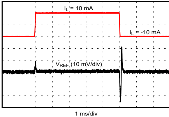
图 6-9. 负载瞬态响应 ( C_{OUT} = 1\text{ }\mu\text{F} )
