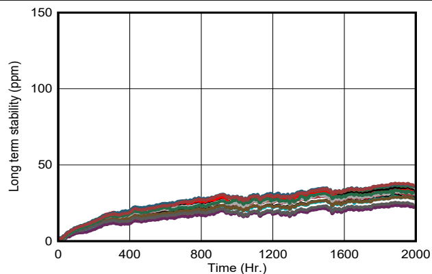
图 6-18. 长期稳定性 (前 2000 小时)
