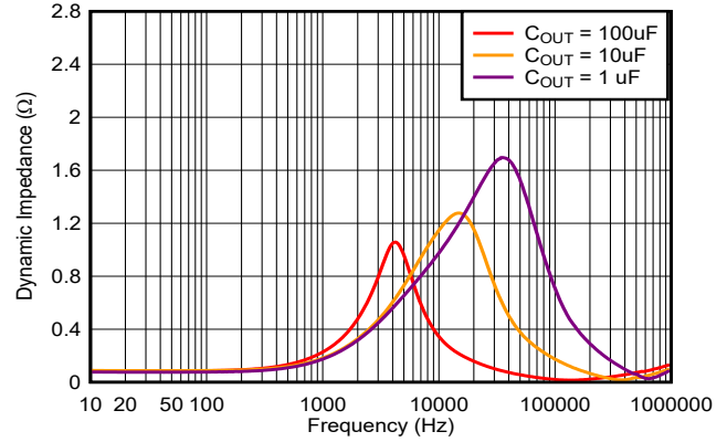
图 6-10. 输出阻抗
