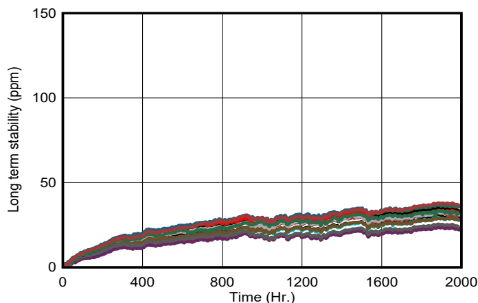
图 7-2. 长期稳定性 SOIC - 2000 小时 ( V_{OUT} )
