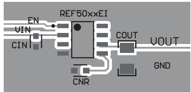
图 11-2. REF50xxEI 布局示例
