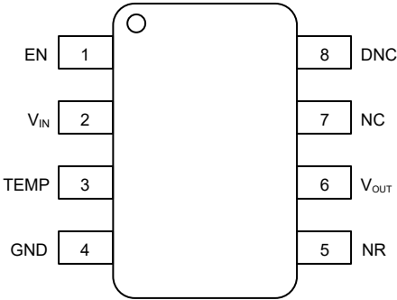
图 5-2. REF50xxEID 封装 8 引脚 SOIC 顶视图
