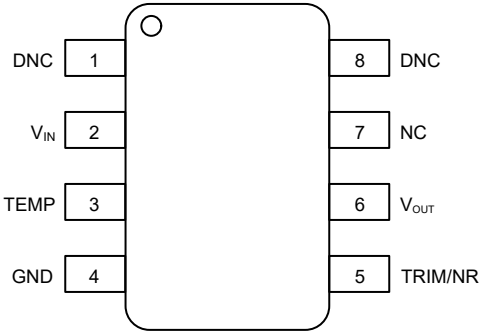
图 5-1. REF50xxAI、REF50xxID、DGK 封装 8 引脚 SOIC、VSSOP 顶视图
