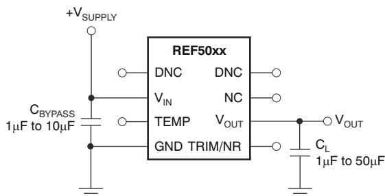
图 8-6. 基本连接
