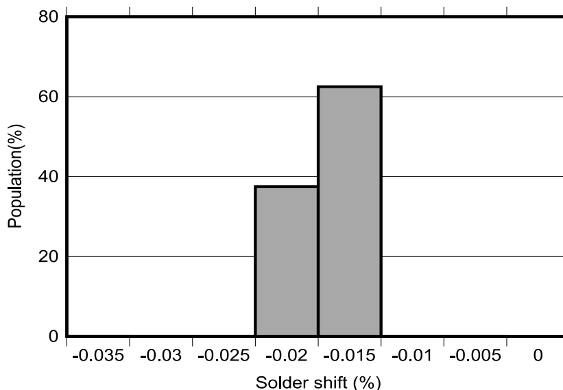
图 7-2. 焊接热移位分布 (%)，REF50xxEI
