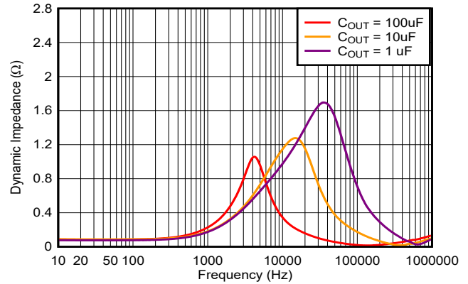
图 6-40. 输出阻抗
