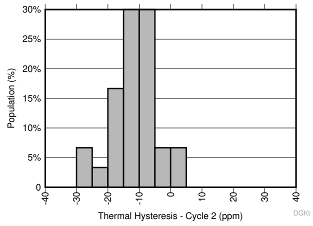
图 9-9. 热迟滞分布 ( V_{REF} ) - DGK 封装 (周期 2)
