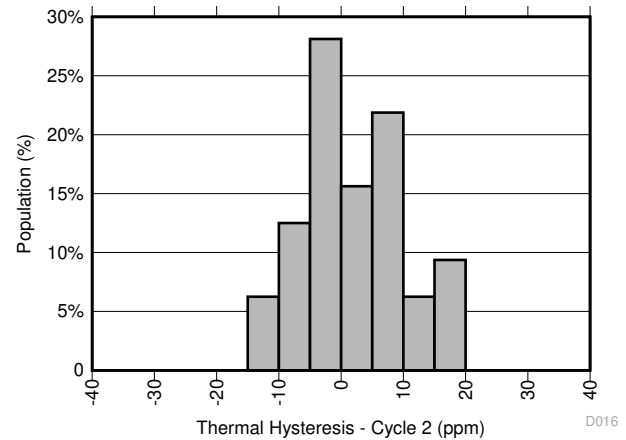
图 9-7. 热迟滞分布 ( V_{REF} ) - DBV 封装 (周期 2)
