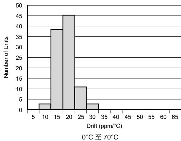
图 6-8. 温漂
