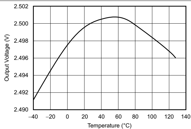
图 6-10. 输出电压与温度间的关系
