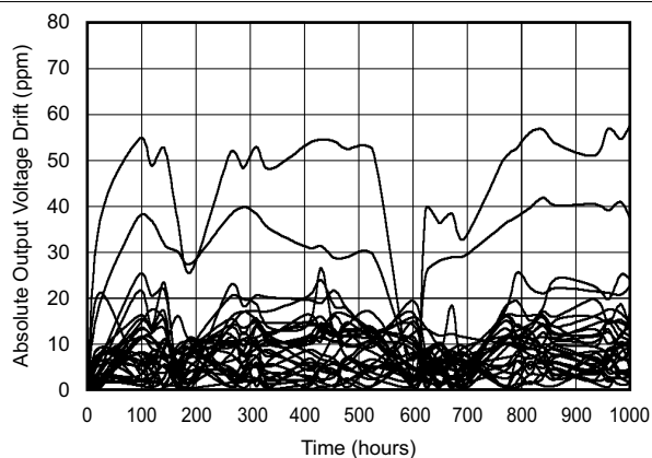
图 6-28. 长期稳定性：0 到 1000 小时
