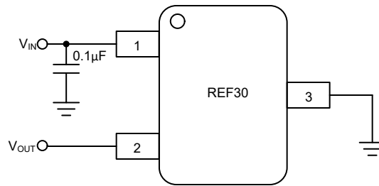
图 8-1. 运行 REF30 的典型连接
