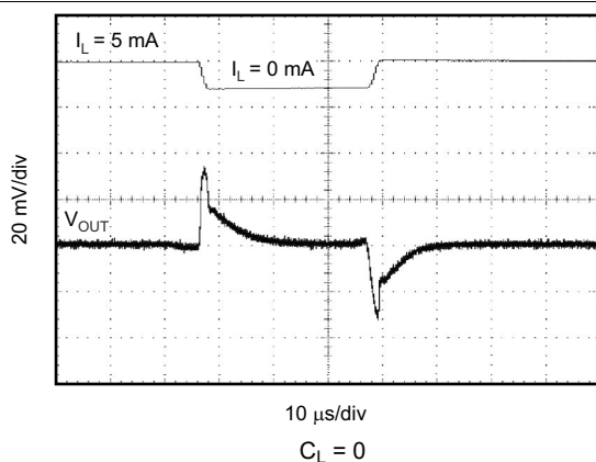
图 6-24. 0mA 至 5mA 负载瞬态
