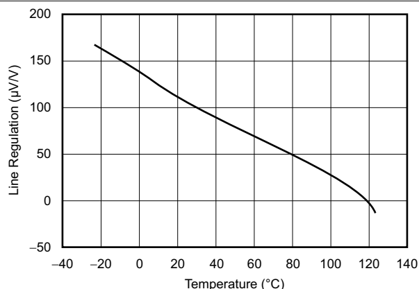
图 6-14. 线路调整率与温度间的关系
