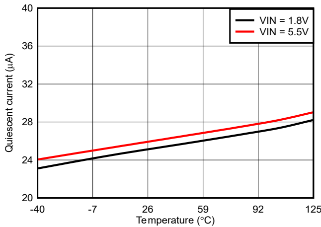
图 6-3. 静态电流与温度间的关系 V_{OUT} = 1.25\text{V}
