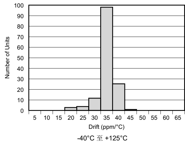
图 6-9. 温漂
