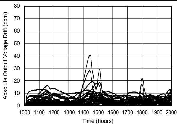
图 6-29. 长期稳定性：1000 到 2000 小时
