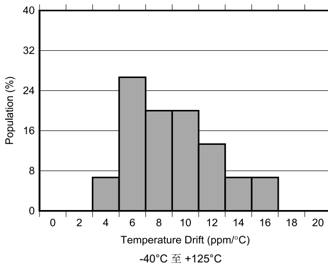
图 6-1. 温漂直方图
