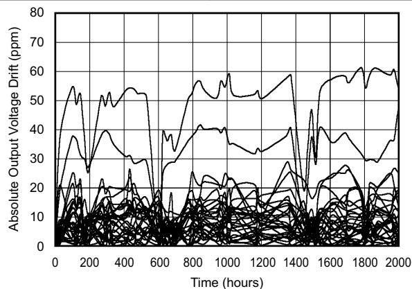
图 6-30. 长期稳定性：0 到 2000 小时
