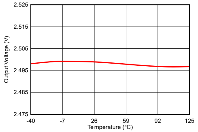
图 6-2. 输出电压与温度间的关系
