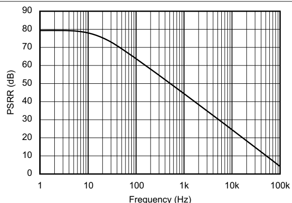
图 6-16. 电源抑制比与频率间的关系
