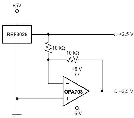
图 7-3. REF3025 与 OPA703 结合使用可产生正和负基准电压。
