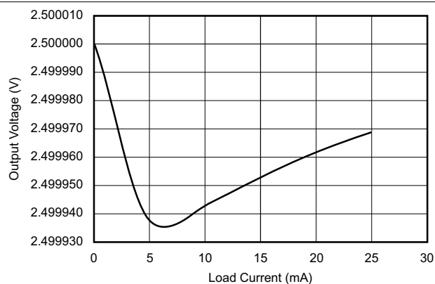
图 6-19. 输出电压与负载电流间的关系
