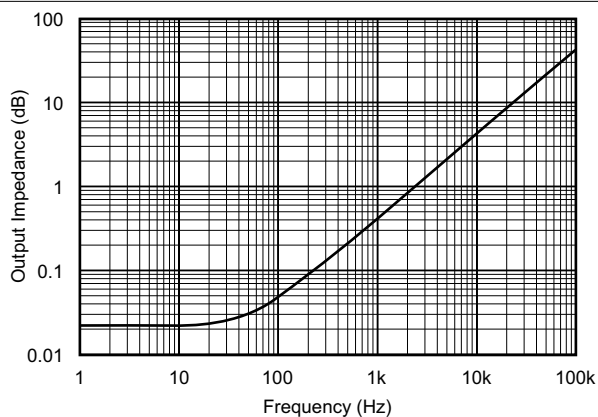
图 6-15. 输出阻抗与频率间的关系
