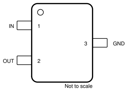
图 5-1. DBZ 封装 3 引脚 SOT-23 顶视图
