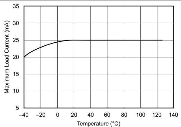
图 6-11. 最大负载电流与温度之间的关系
