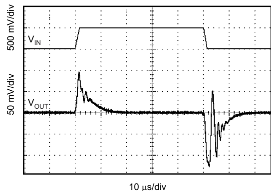
图 6-22. 线路瞬态响应
