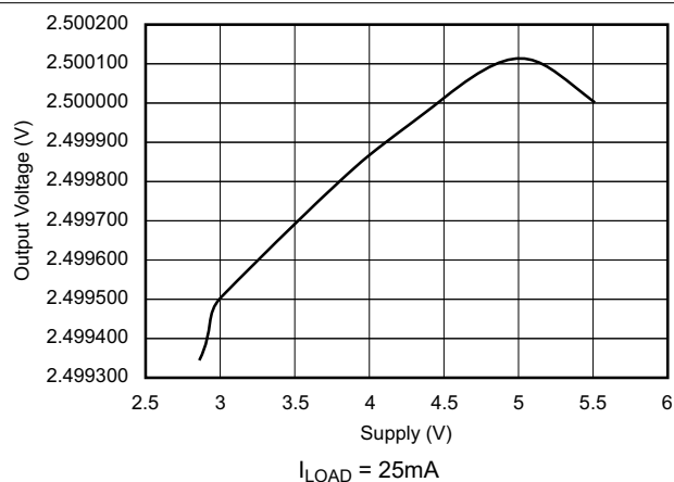
图 6-18. 输出电压与电源电压之间的关系
