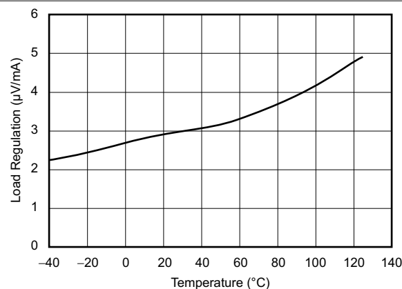
图 6-12. 负载调节与温度之间的关系
