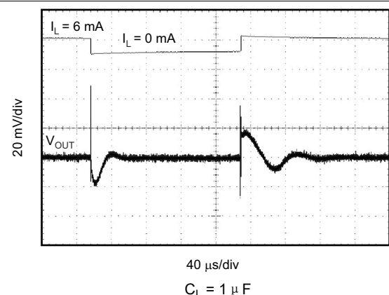
图 6-25. 1mA 至 6mA 负载瞬态
