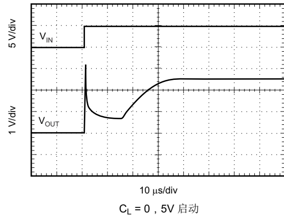
图 6-21. 阶跃响应
