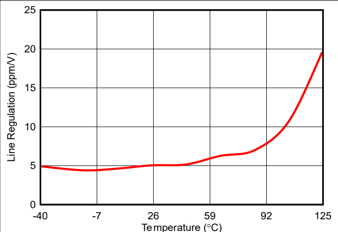
图 6-6. 线路调整率与温度间的关系
