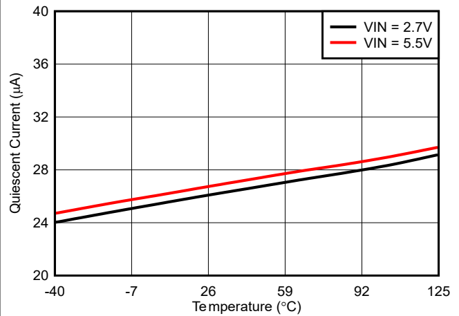
图 6-4. 静态电流与温度间的关系 V_{OUT} = 2.5\text{V}
