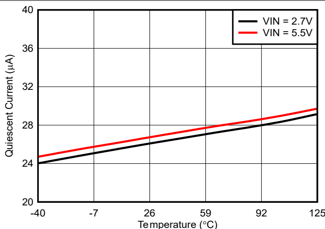
图 6-5. 静态电流与温度间的关系 V_{OUT} = 3\text{V}
