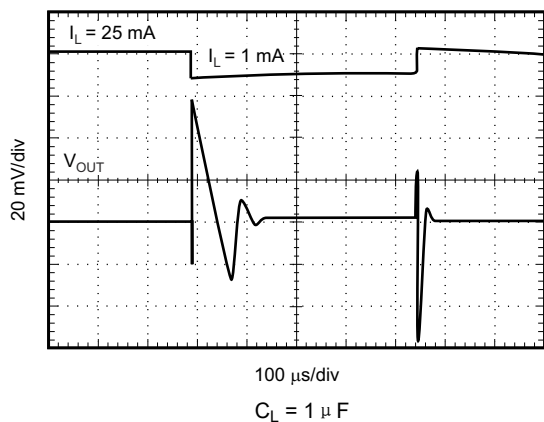
图 6-26. 1mA 至 25mA 负载瞬态
