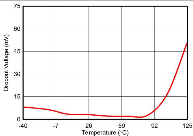
图 6-7. 压降电压与温度间的关系
