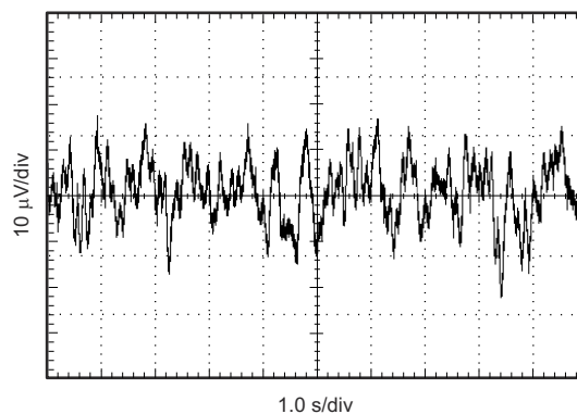
图 6-27. 0.1Hz 至 10Hz 噪声
