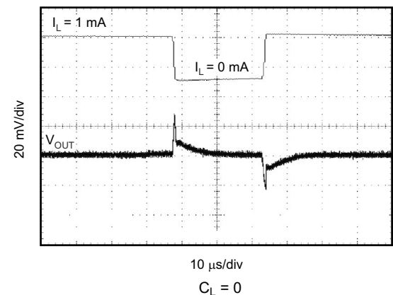
图 6-23. 0mA 至 1mA 负载瞬态
