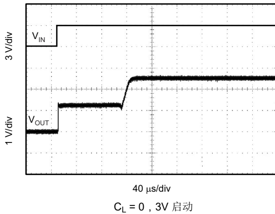
图 6-20. 阶跃响应
