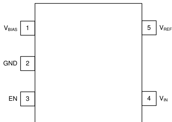
图 6-1. DDC Package SOT23-5 (Top View)
