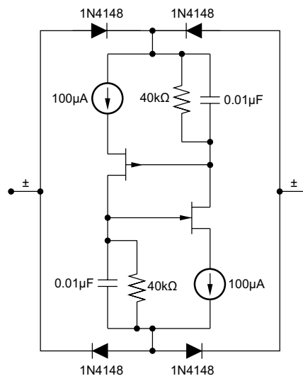
(d) Bidirectional 200µA cascoded current source.
