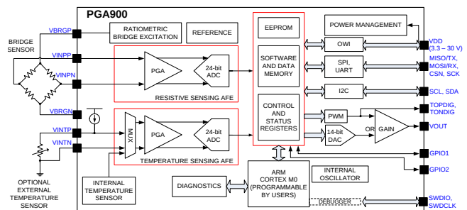
PGA900 简化方框图
