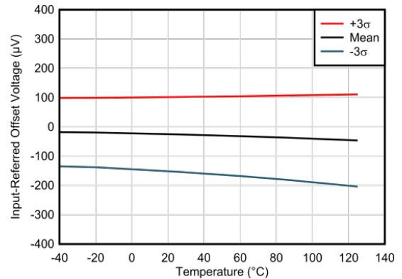
图 6-4. 失调电压 (RTI) 与温度间的关系
