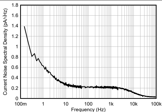
图 6-32. 电流噪声频谱密度与频率间的关系
