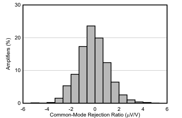
图 6-16. CMRR 分布
