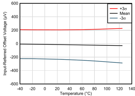
图 6-3. 失调电压 (RTI) 的分布
