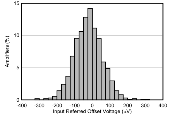
图 6-2. 失调电压 (RTI) 的分布
