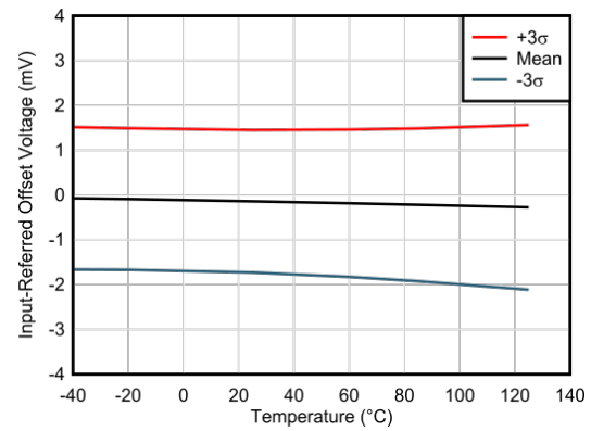
图 6-2. 失调电压 (RTI) 的分布
