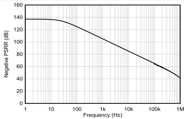
图 6-13. PSRR 分布图
