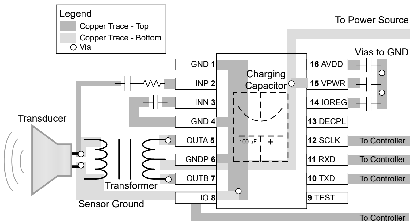
图 8-9. PGA460 布局示例
